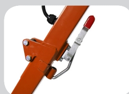
Poignée de manœuvre pliable pour faciliter le transport
